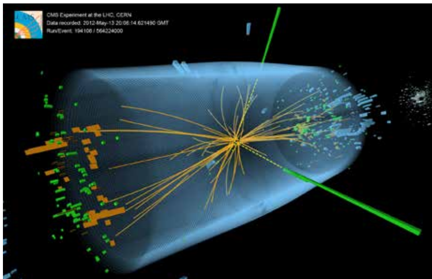
Data från CMS-experimentet vid CERN. Bild: © 2013 CERN, for the benefit of the CMS Collaboration. Image credit: Thomas McCauley and Lucas Taylor.
